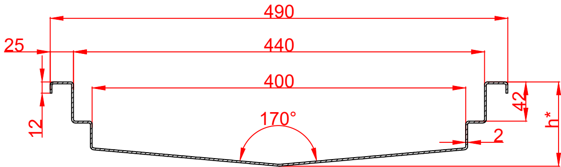
A-A (1:4)
